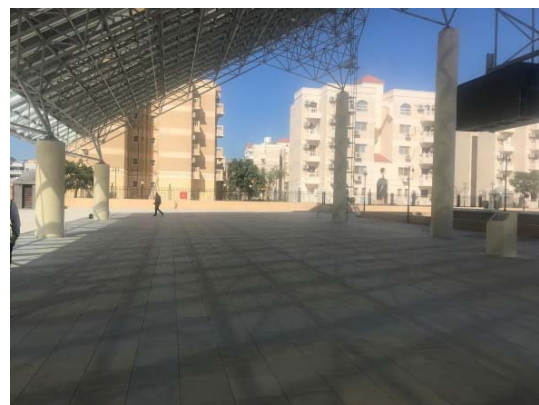
エントランス広場となるアトリウム棟には採光を考慮しシースルー型アモルファス系太陽電池モジュールを設置
