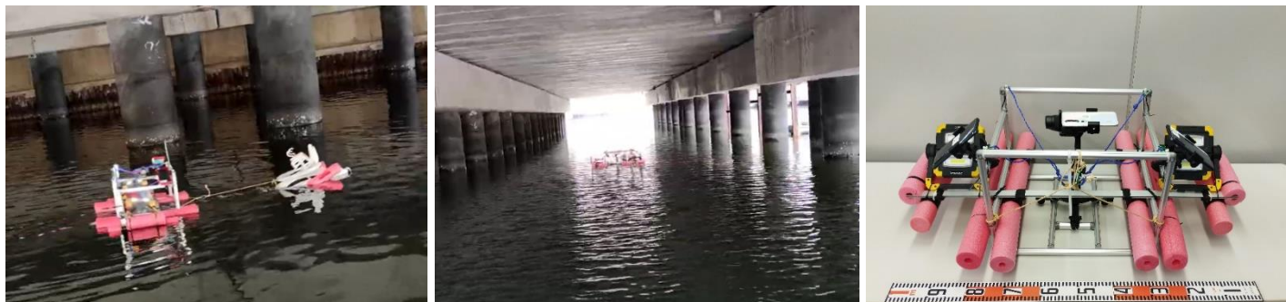
【海上で水平画像を容易に撮影できるようジンバルカメラを搭載した水上ドローン】
