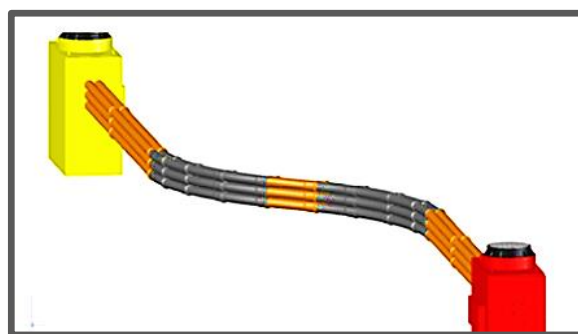
電線共同溝 管路詳細 3D モデル
