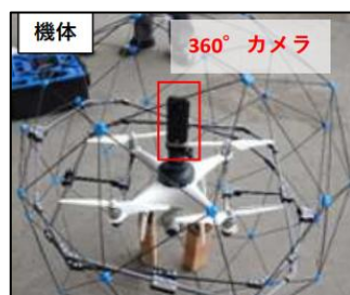
①球体ガードと 360° カメラ搭載ドローン (鋼橋主桁間等撮影)
