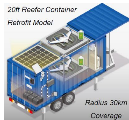
コンテナ型自動発着ポート イメージ図 画像提供：エアロセンス株式会社
